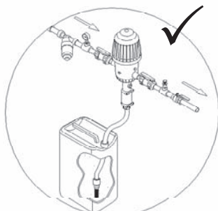
Installation correcte
